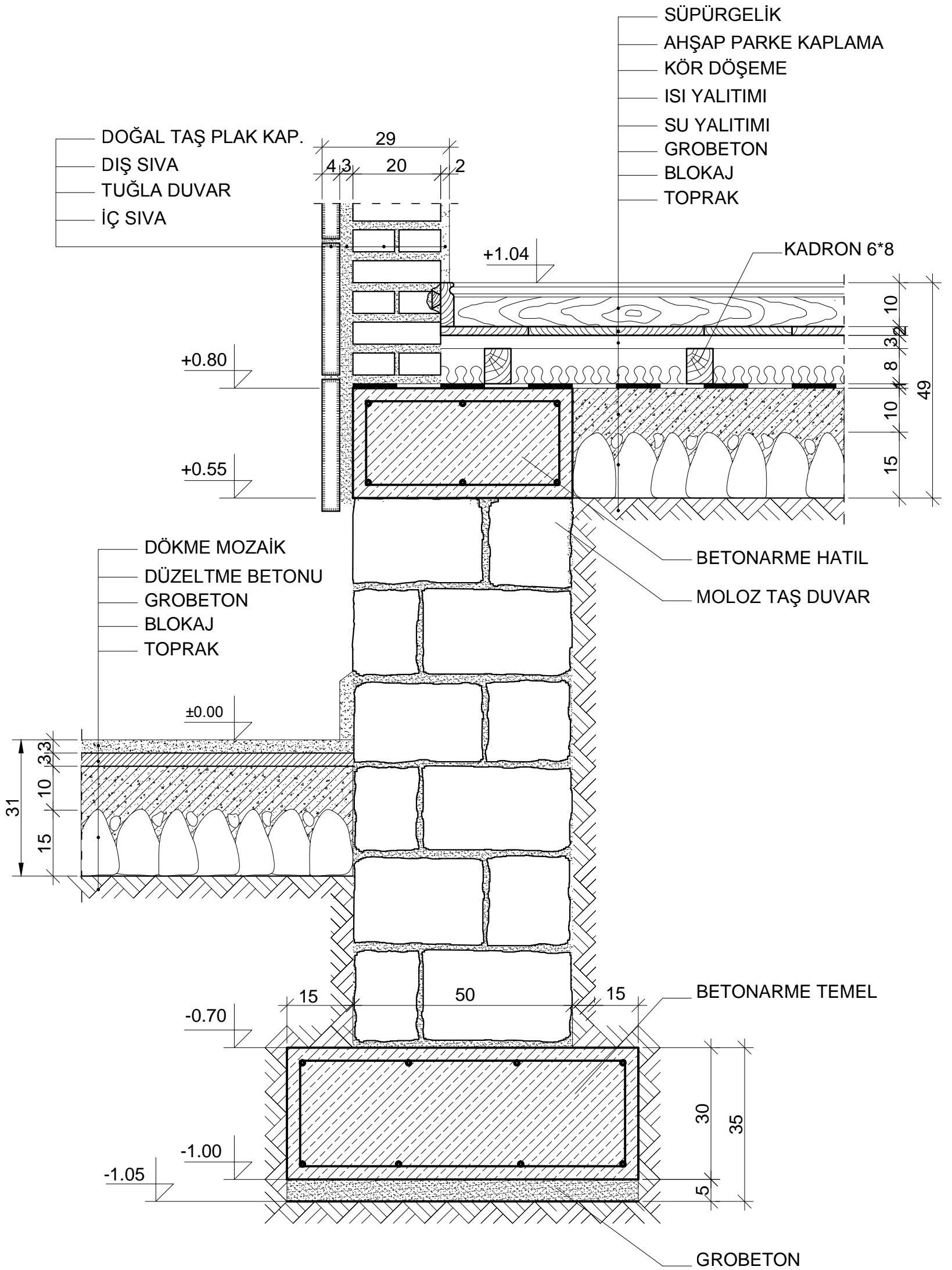
TAŞ TEMEL SİSTEM DETAYI Ö:1/10
