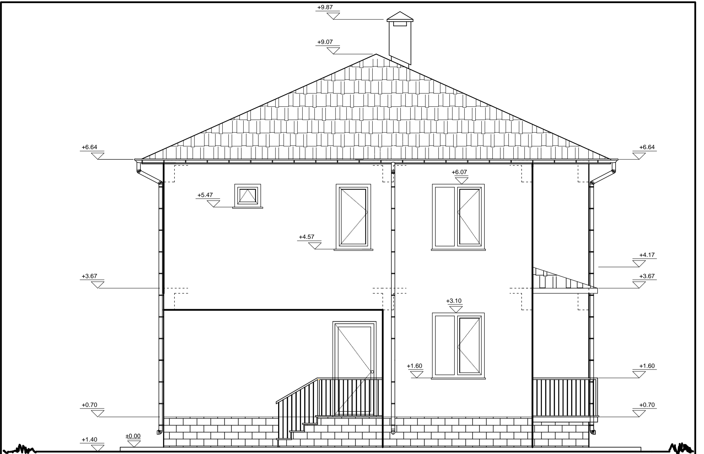
ÖN GÖRÜNÜŞ Ö:1/50
