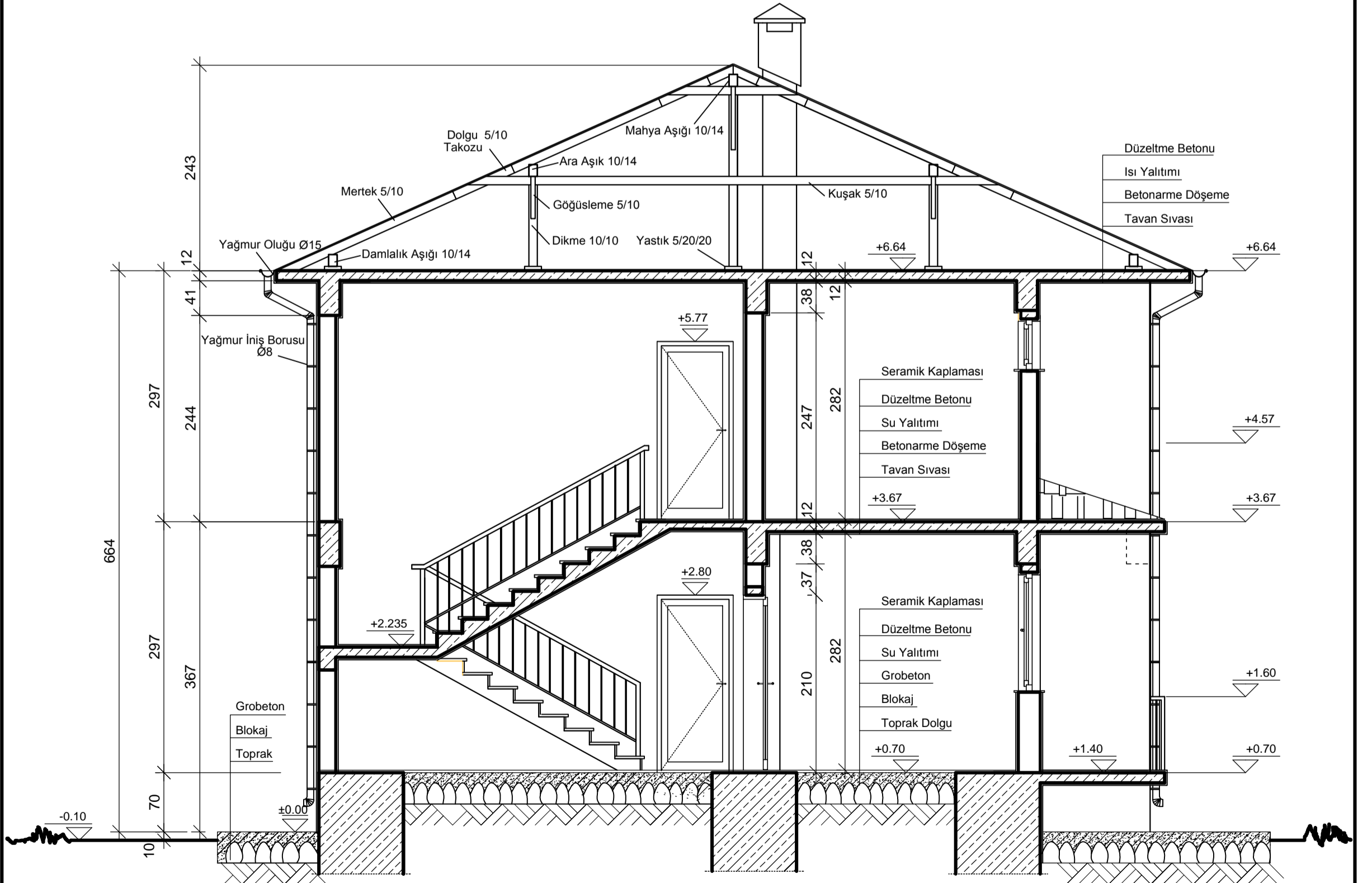
A-A KESİTİ Ö:1/50
