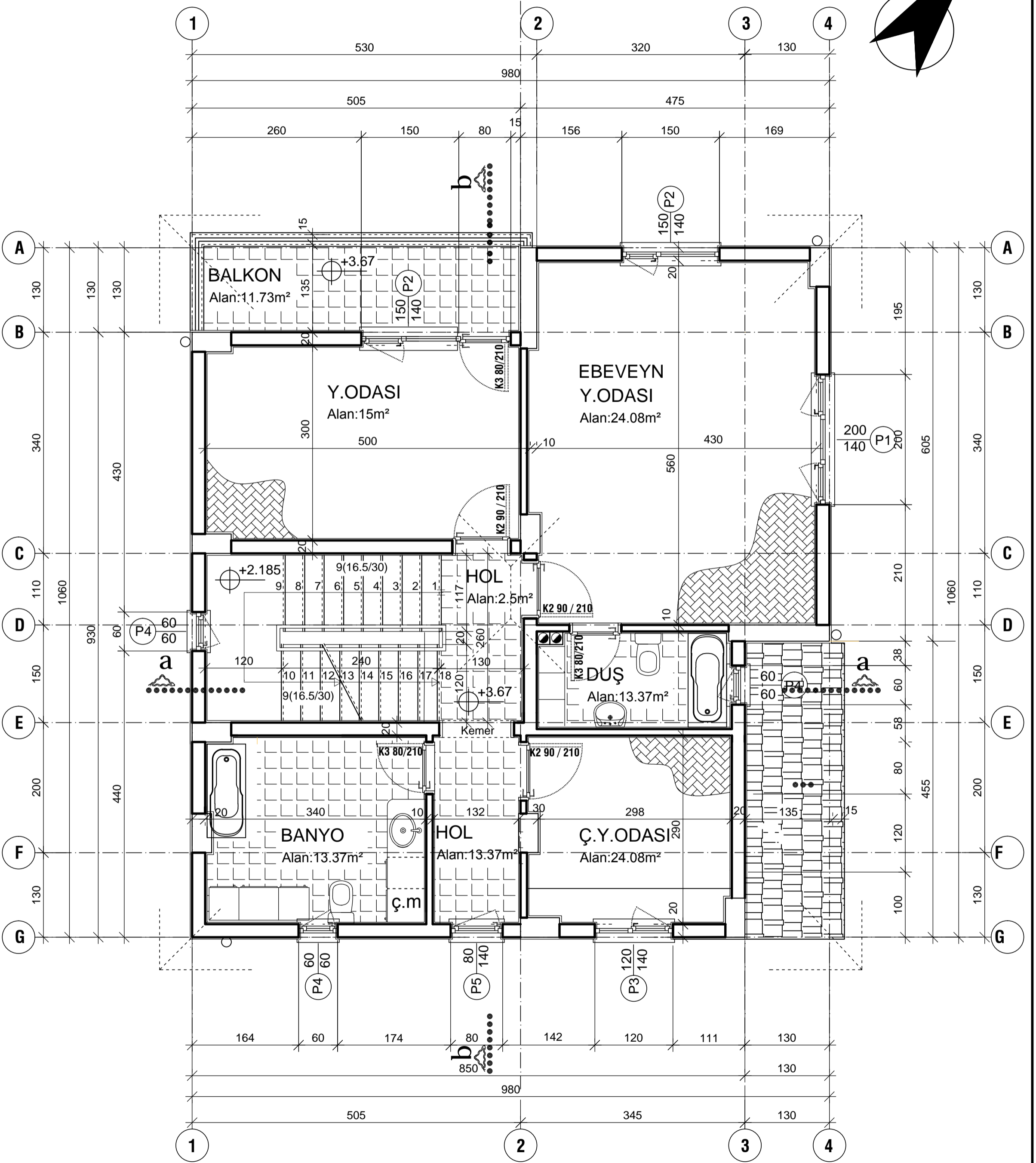
ÜST KAT PLANI Ö:1/50
