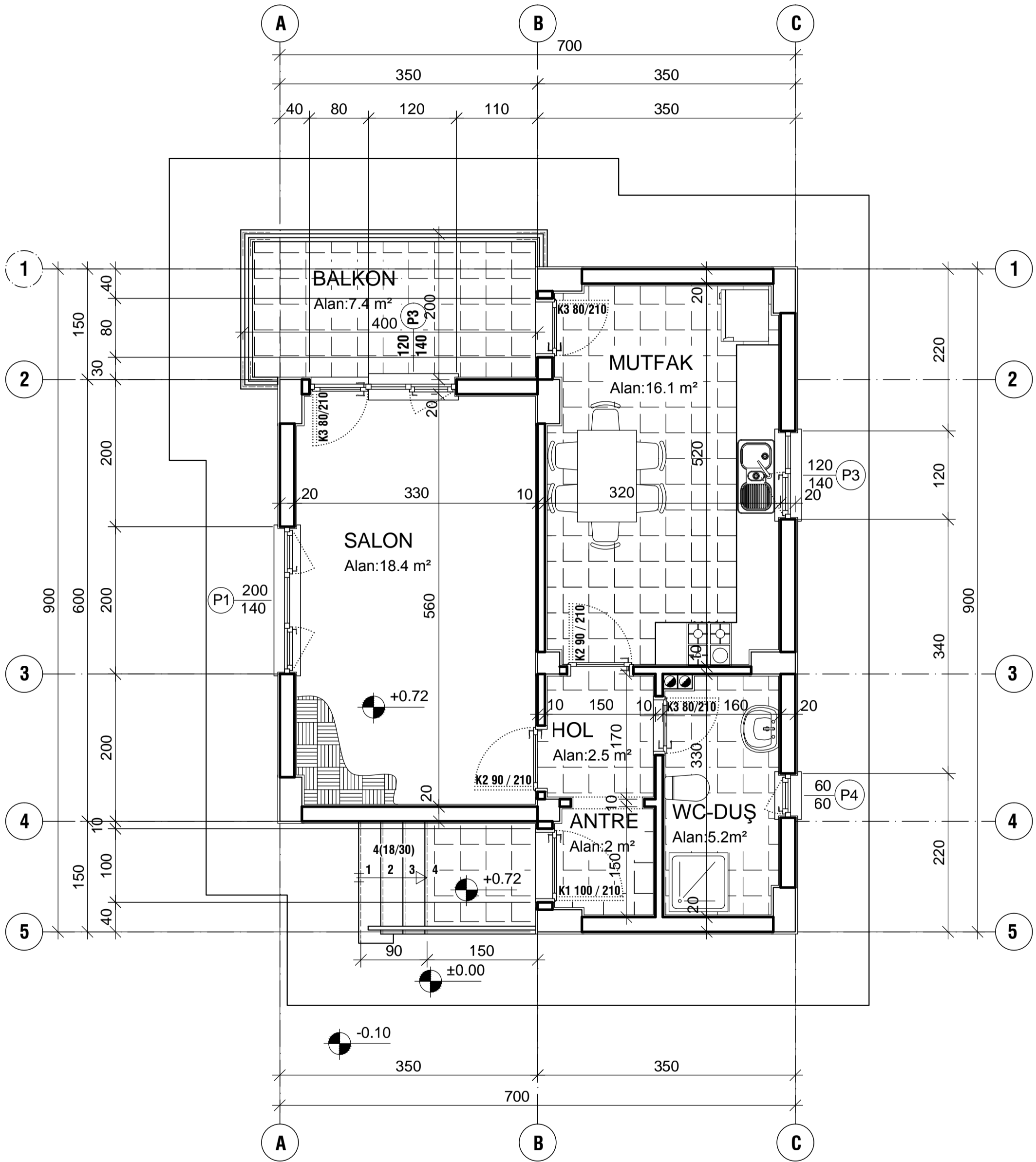
ZEMİN KAT PLANI Ö:1/50
