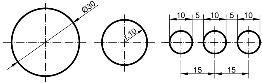
DAİRELERİN ÖLÇÜLENDİRİLMESİ Ö:1/10
