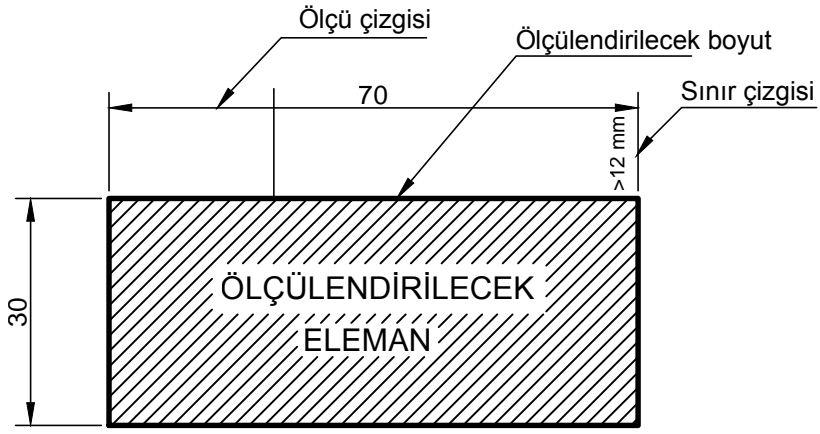
BİR BOYUTUN ÖLÇÜLENDİRİLMESİ Ö:1/10
