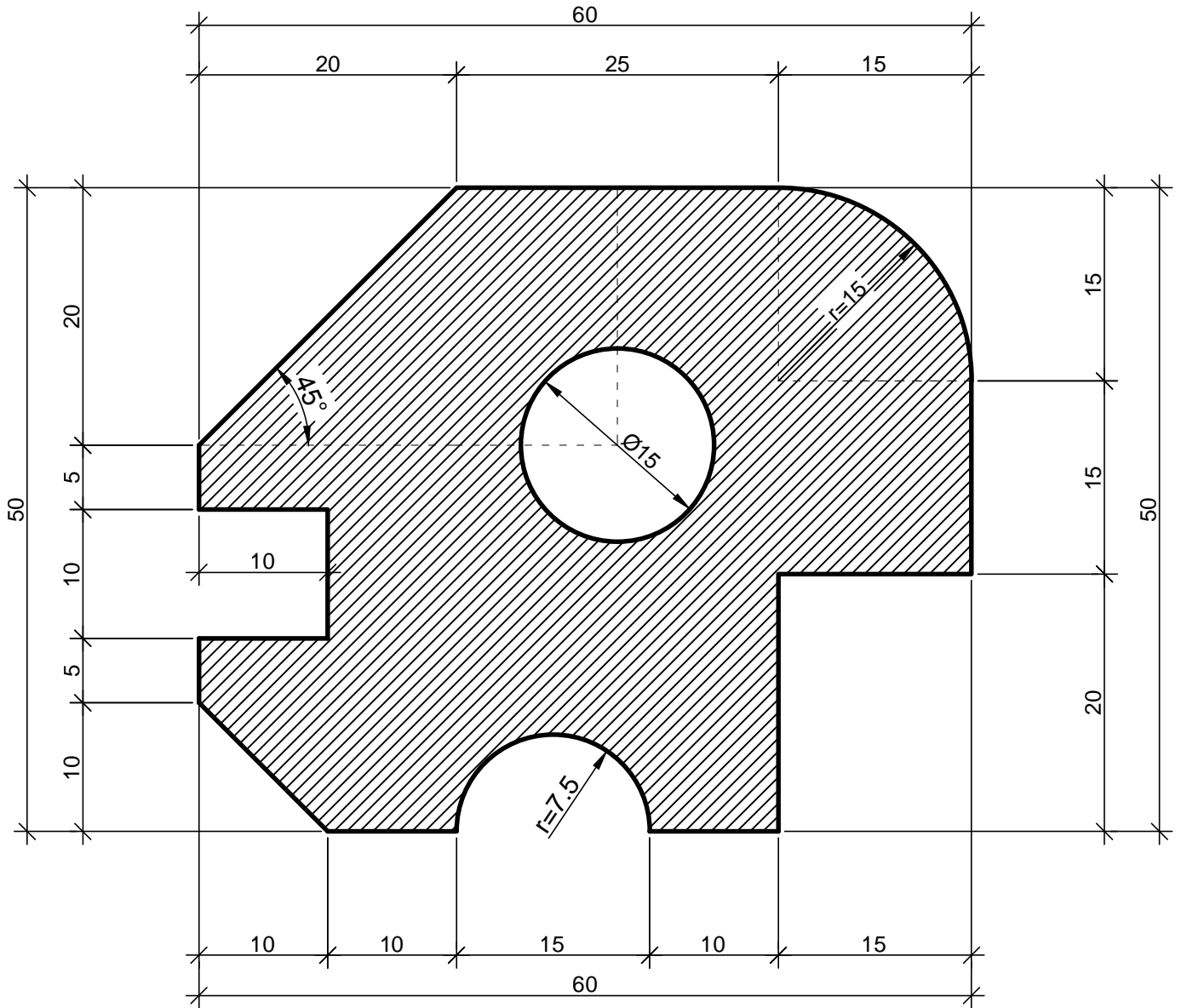
CİSMİN ÖLÇÜLENDİRİLMESİ Ö:1/5
