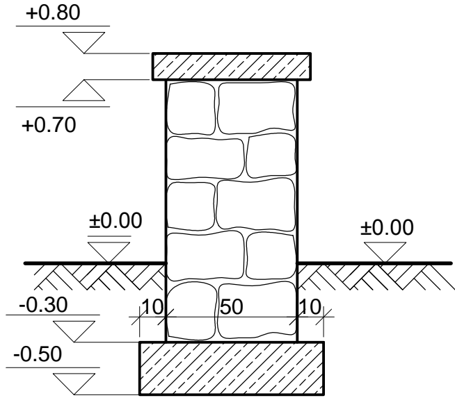
A-A KESİTİ Ö:1/20
