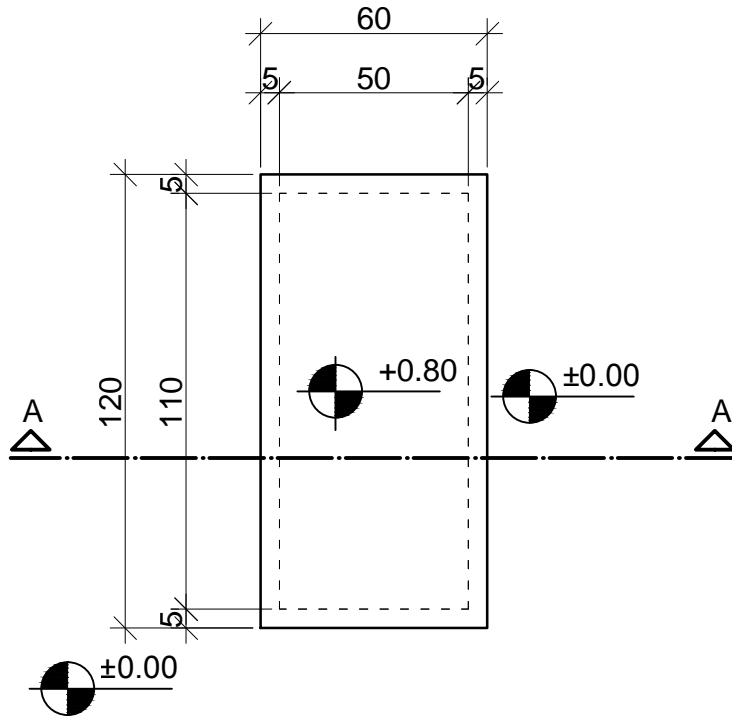
TAŞ DUVAR PLANI Ö:1/20
