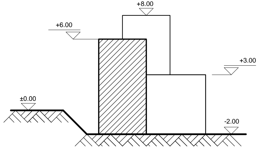
A-A KESİTİ Ö:1/200
