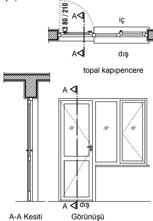
PENCERELER (Kesit ve Görünüşte)
