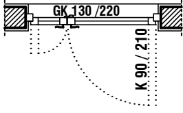
130'luk bina kapısı
