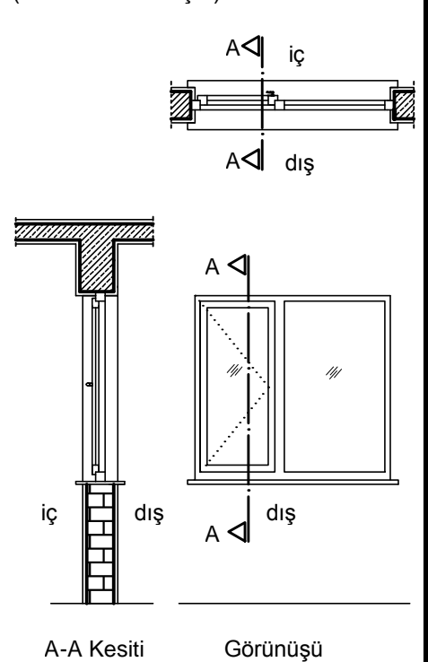
PENCERELER (Kesit ve Görünüşte)
