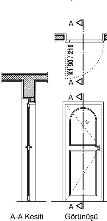
KAPILAR (Kesit ve Görünüşte)
