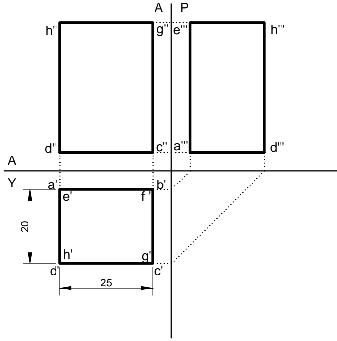
DİKDÖRTGENLER PRİZMASININ İZDÜŞÜMLERİ
