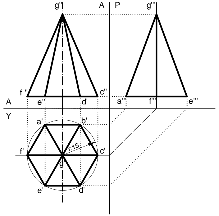
ALTIGEN PRAMİDİN İZDÜŞÜMLERİ
