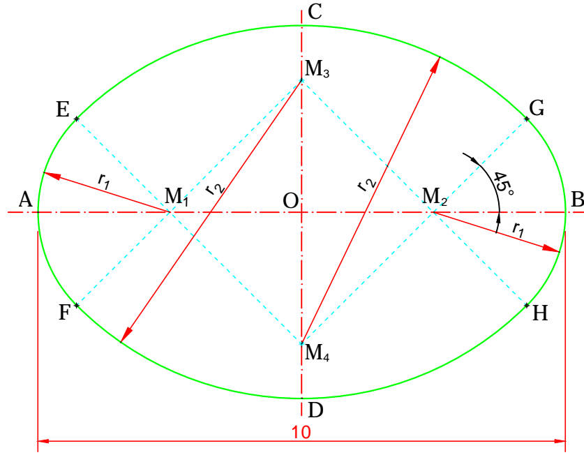
DÖRT MERKEZLİ ELİPS ÇİZİMİ
