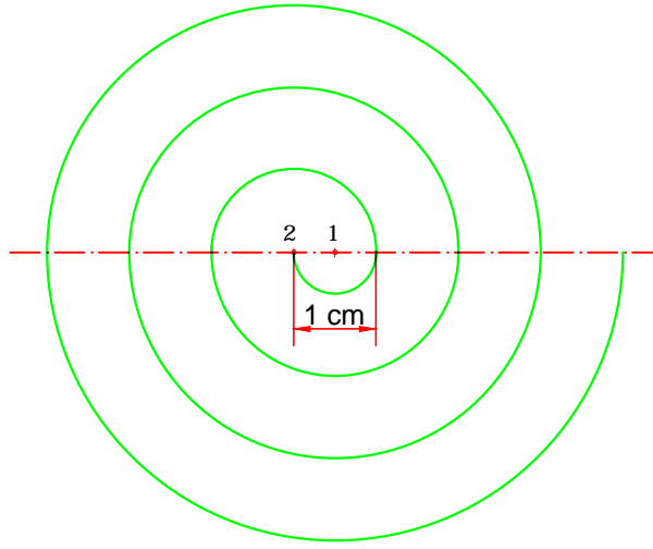
İKİ MERKEZLİ SPİRAL ÇİZİMİ
