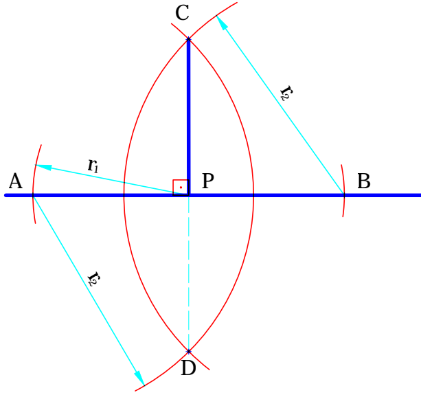
DOĞRU ÜZERİNDEKİ P NOKTASINDAN DİK ÇIKMAK
