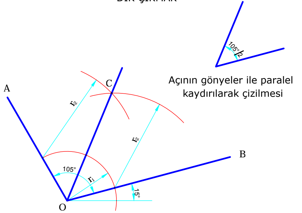
105° LİK AÇIYI İKİ EŞİT PARÇAYA BÖLMEK
