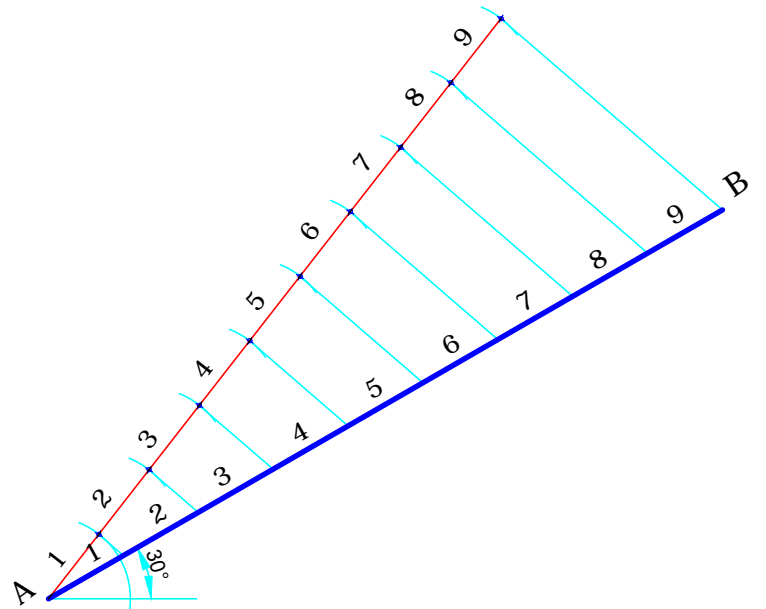
BİR DOĞRU PARÇASINI DOKUZ EŞİT PARÇAYA BÖLMEK
