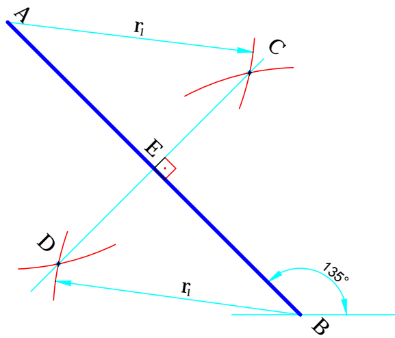
BİR DOĞRU PARÇASINI İKİ EŞİT PARÇAYA BÖLMEK
