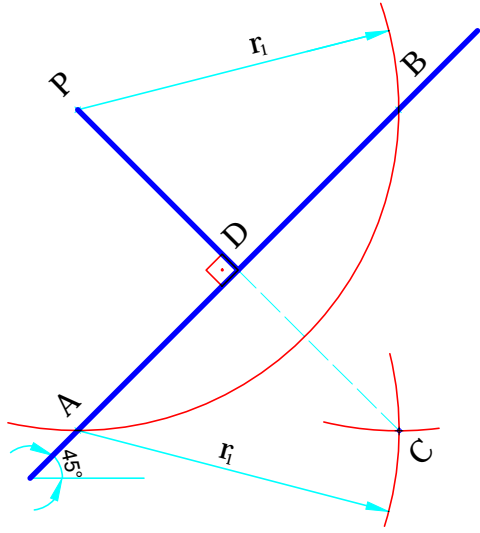
DOĞRUNUN DIŞINDAKİ P NOKTASINDAN DİK İNMEK
