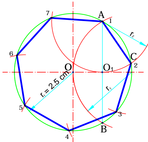
ÇEMBER İÇERİSİNE DÜZGÜN YEDİGEN ÇİZİMİ
