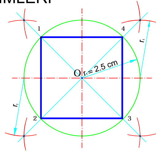
ÇEMBER İÇERİSİNE DÜZGÜN DÖRTGEN ÇİZİMİ
