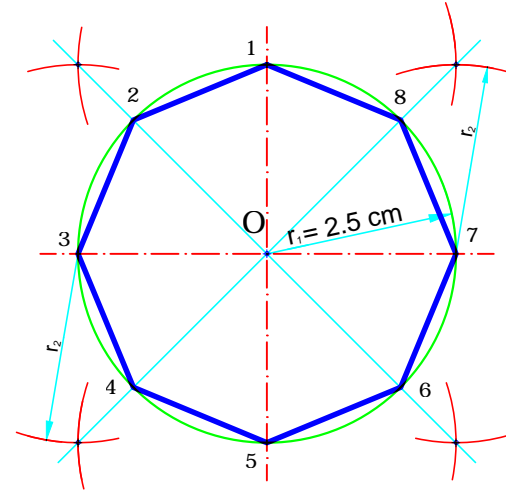
ÇEMBER İÇERİSİNE DÜZGÜN SEKİZGEN ÇİZİMİ
