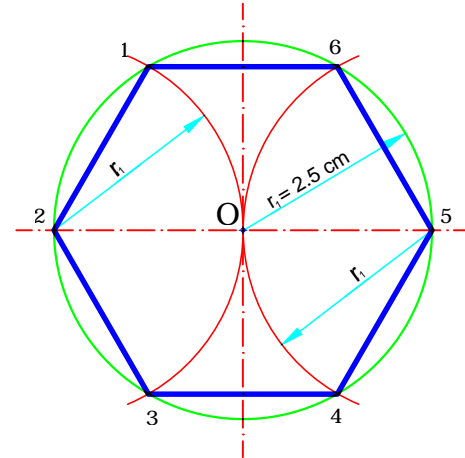
ÇEMBER İÇERİSİNE DÜZGÜN ALTIGEN ÇİZİMİ
