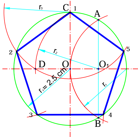
ÇEMBER İÇERİSİNE DÜZGÜN BEŞGEN ÇİZİMİ
