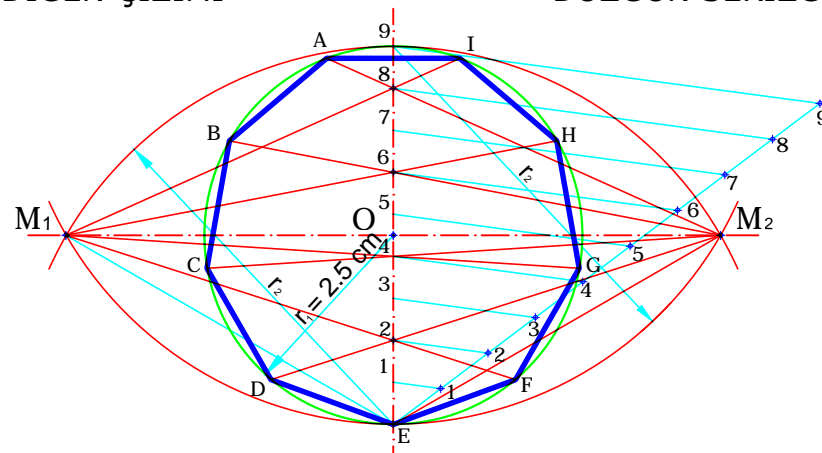
ÇEMBER İÇERİSİNE GENEL METOD İLE DÜZGÜN DOKUZGEN ÇİZİMİ
