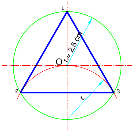
ÇEMBER İÇERİSİNE DÜZGÜN ÜÇGEN ÇİZİMİ
