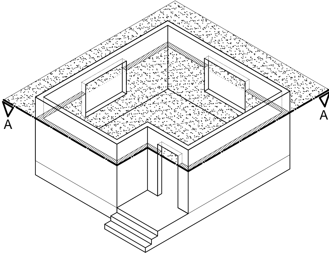
BİNANIN PERSPEKTİFİ Ö:1/100
