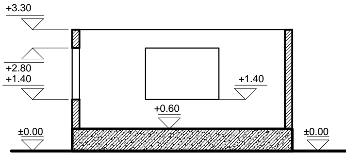
B-B KESİTİ Ö:1/100
