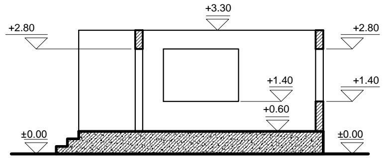
C-C KESİTİ Ö:1/100
