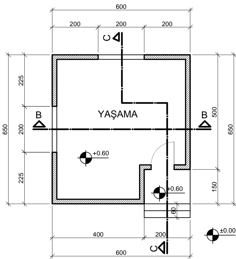
A-A KESİTİ (PLAN) Ö:1/100
