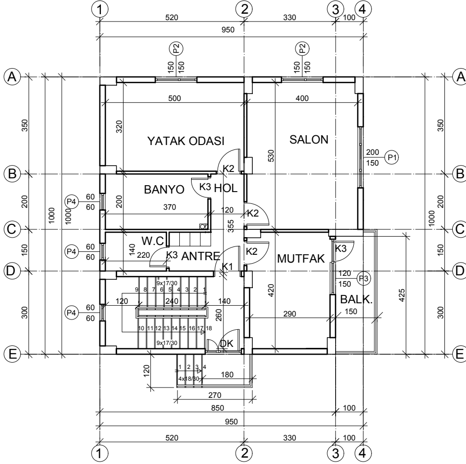
ZEMİN KAT PLANI Ö:1/50
